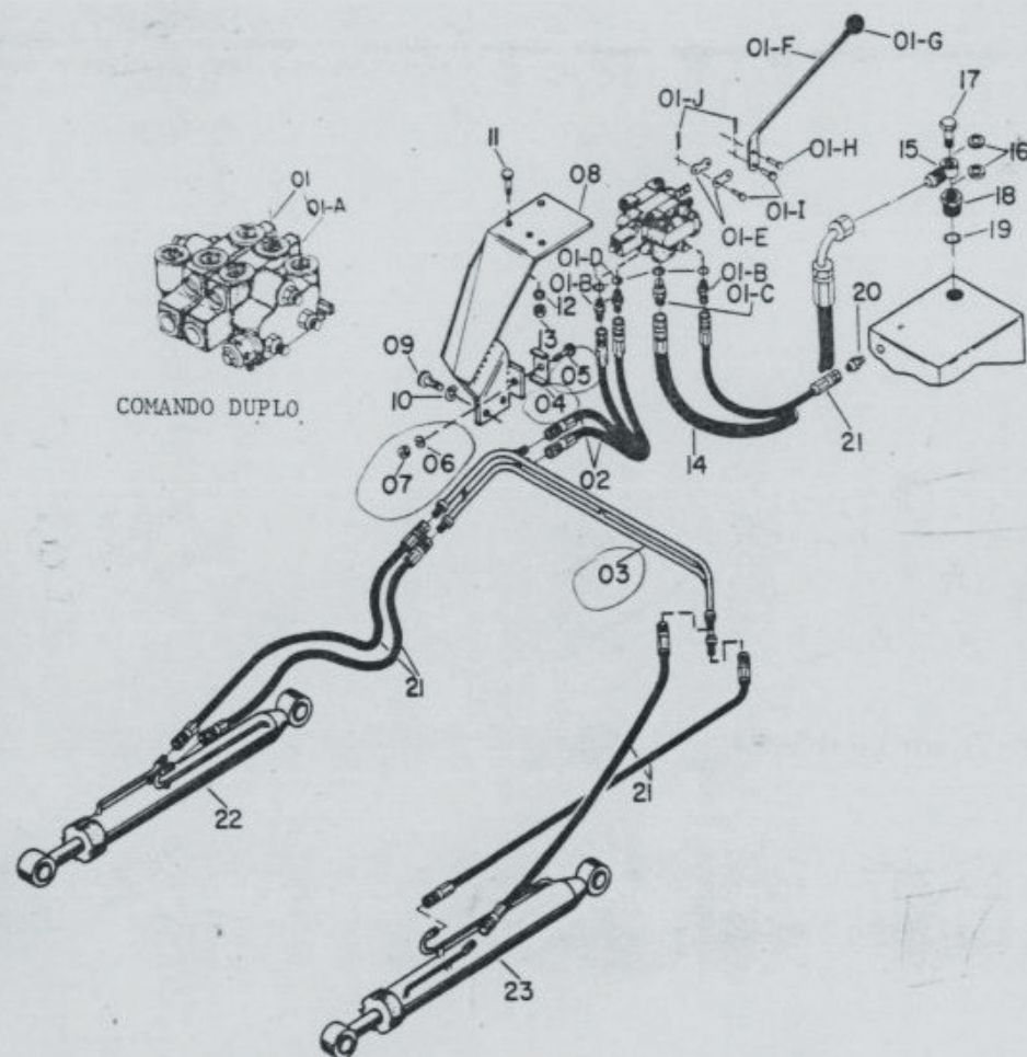
Cilindro Hidráulico (item 22/23) Vide Folha nº 005
