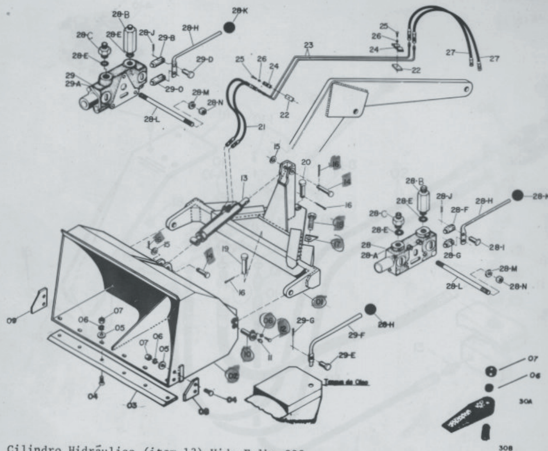
Cilindro Hidráulico (item 13) Vide Folha 008
