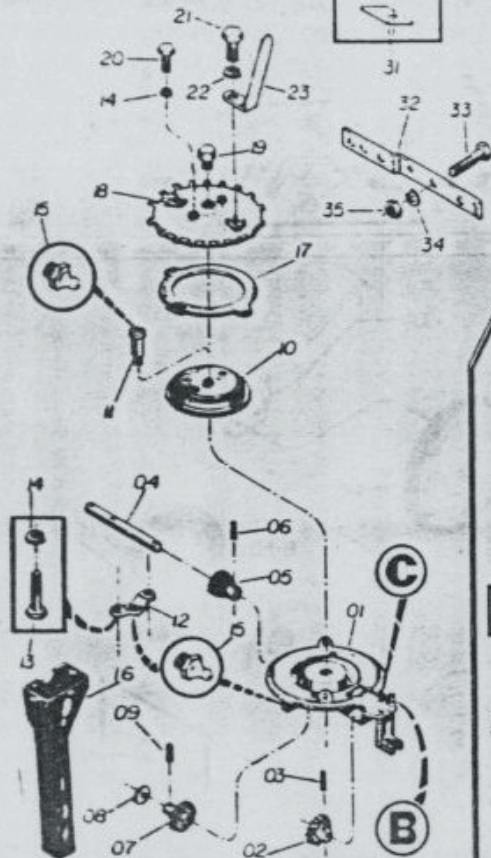
SISTEMA DE SEMENTE - ALGODÃO EM LINTER
