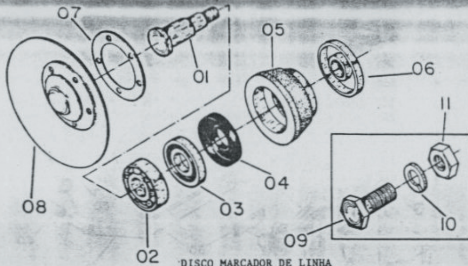
DISCO MARCADOR DE LINHA
