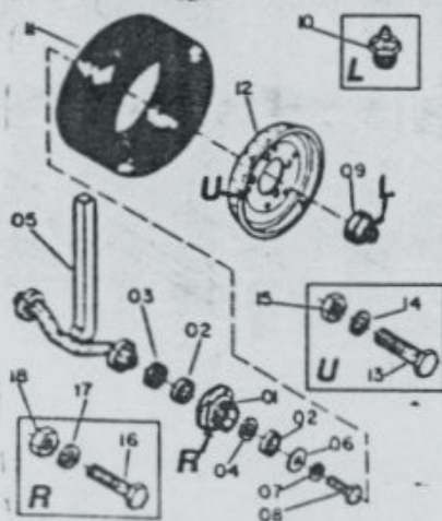
RODA DE PROFUNDIDADE
