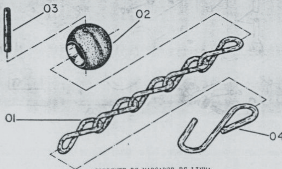
CORRENTE DO MARCADOR DE LINHA
