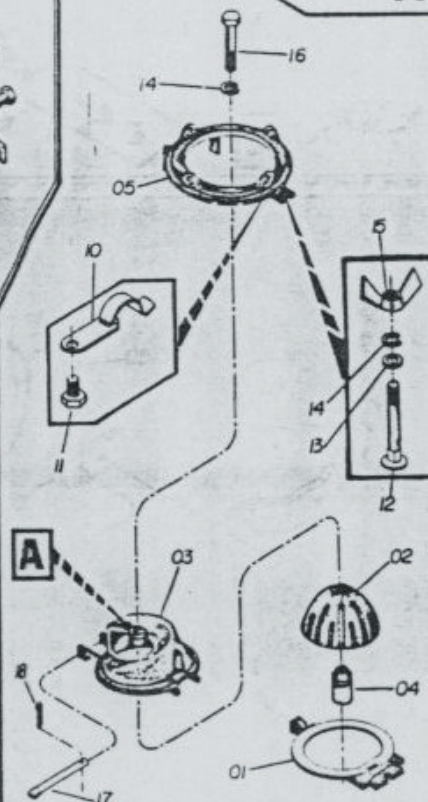
SISTEMA DE SEMENTE - AMENDOIM
