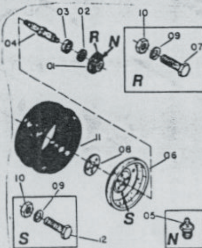
RODA COMPACTADORA
