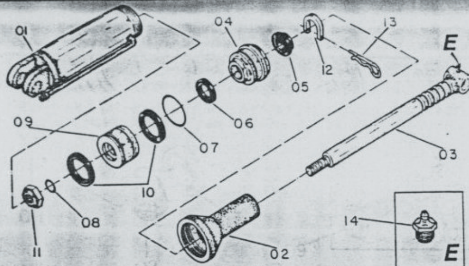
CIL. HIDR. Ø 50,8 x Ø 101 x 617 x 180
