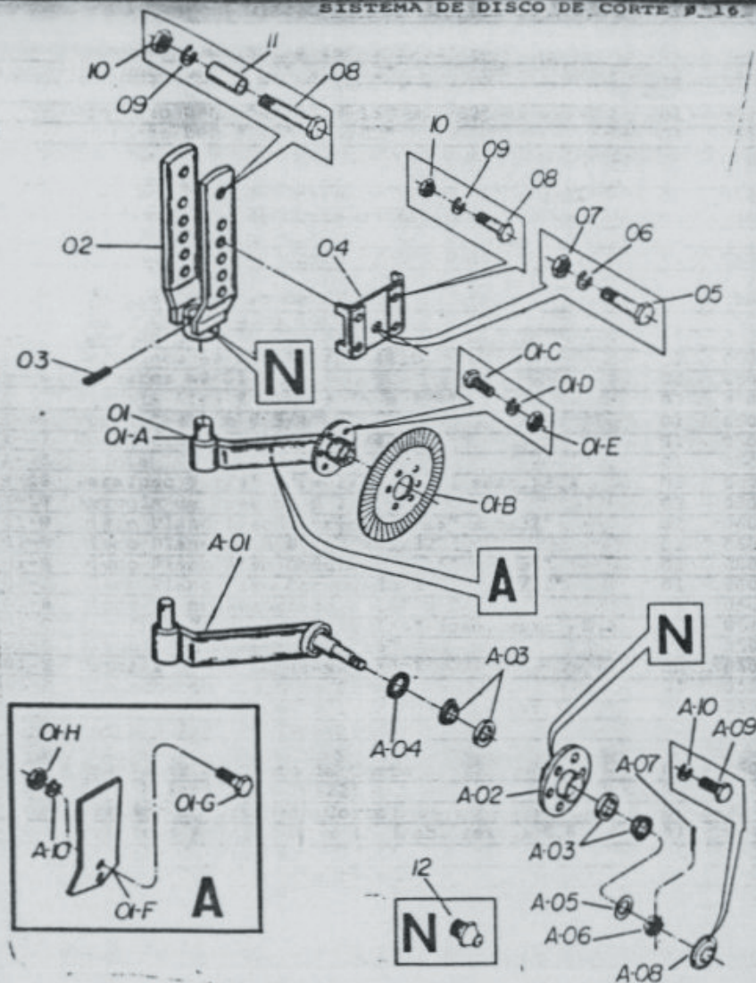
SISTEMA DE DISCO DE CORTE Ø 16"
