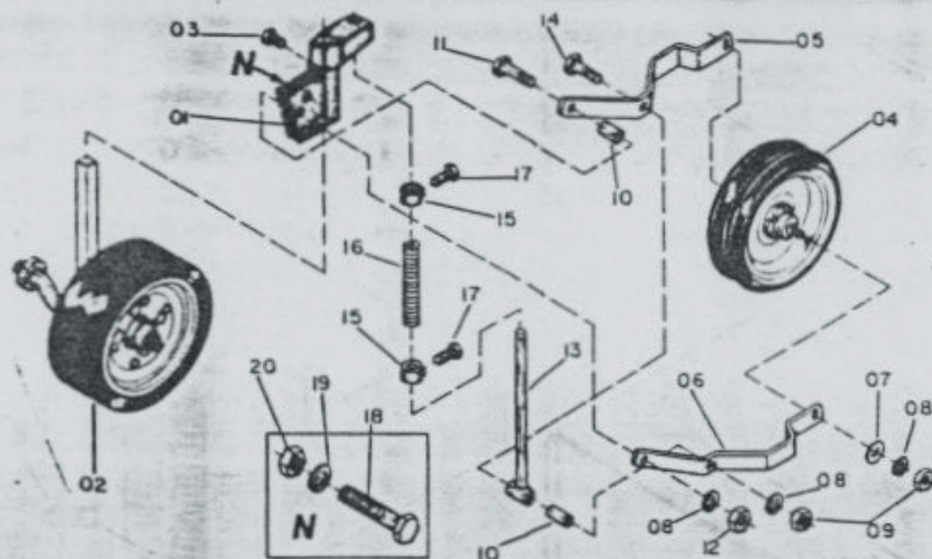
SISTEMA DE COMPACTAÇÃO E RODA DE PROFUNDIDADE
