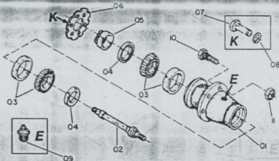
SISTEMA DE RODAGEM S/ PNEU
