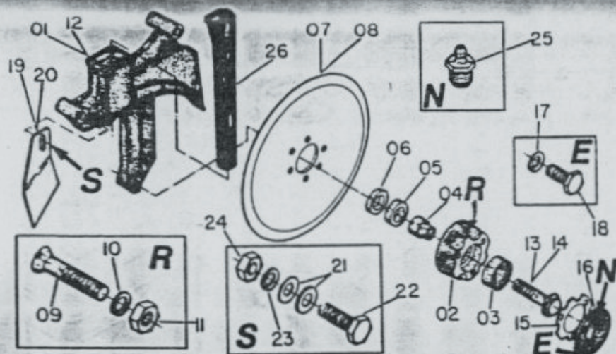
DISCO DUPLO DESENCONTRADO (SEMENTE)
