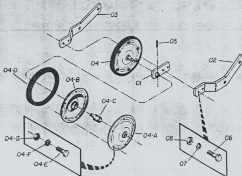
SISTEMA DE COMPACTAÇÃO EM "V"
