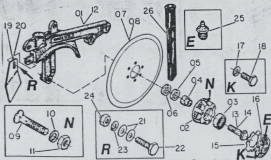
DISCO DUPLO DESENCONTRADO (ADUBO)
