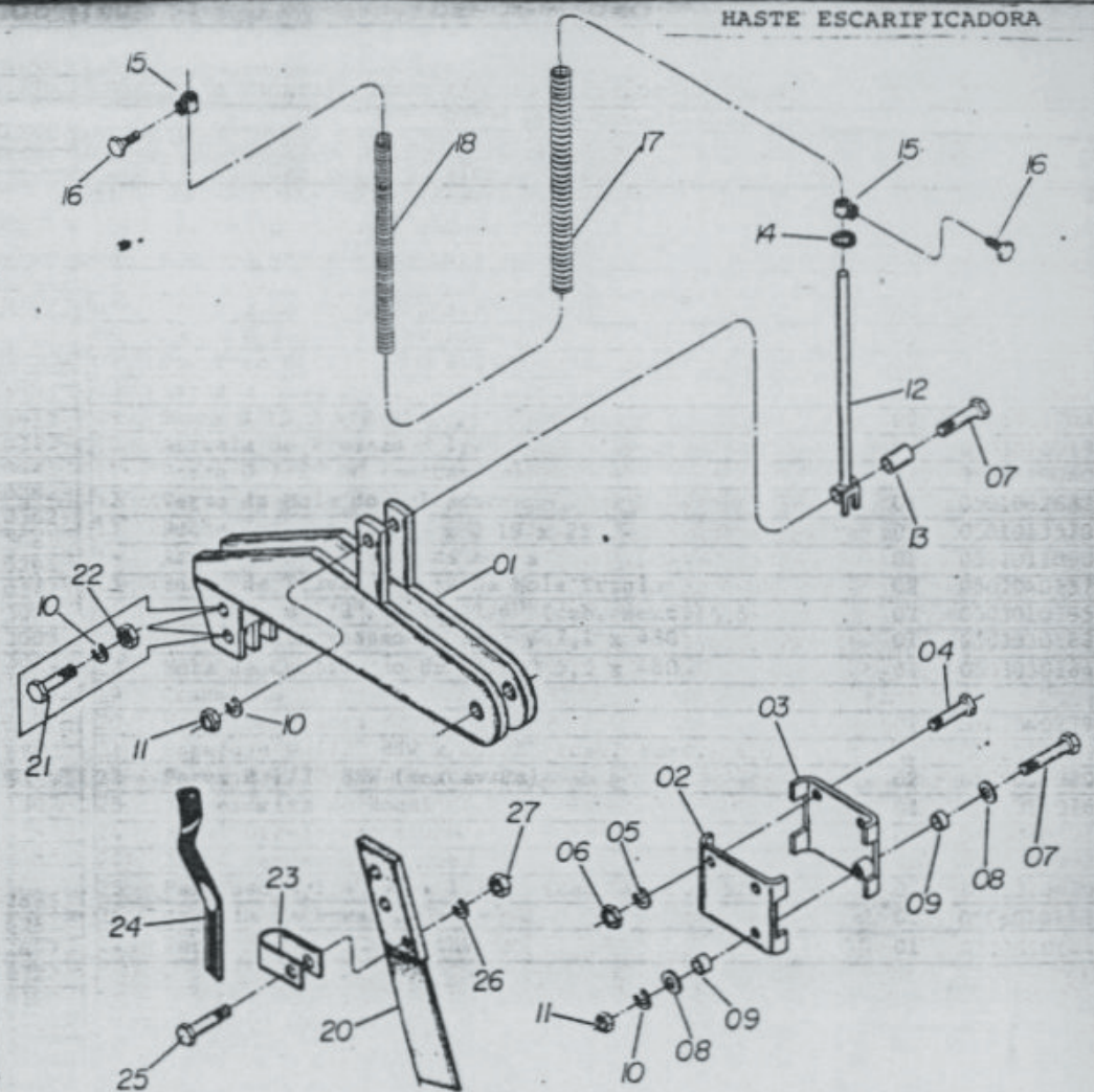
HASTE ESCARIFICADORA
